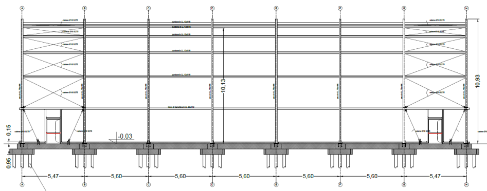
SEZIONE 03 scala 1.100
