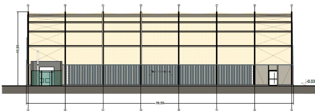
SEZIONE 03 scala 1.100
