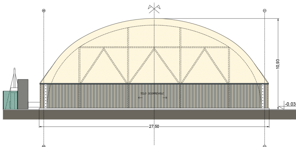
PROSPETTO OVEST scala 1.100
